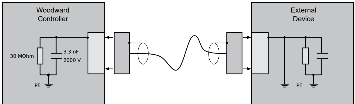
Fig. 79: Préparation du blindage (élément RC interne)
