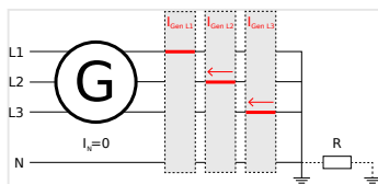
Fig. 135: Défaut à la terre du générateur - schéma
