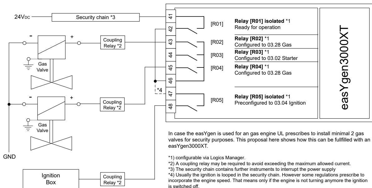
Fig. 70: Contrôle des vannes de gaz conformément à la réglementation UL
