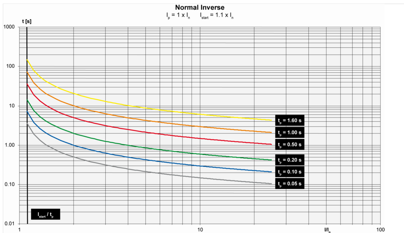
Fig. 129: Caractéristique « inverse normale »
