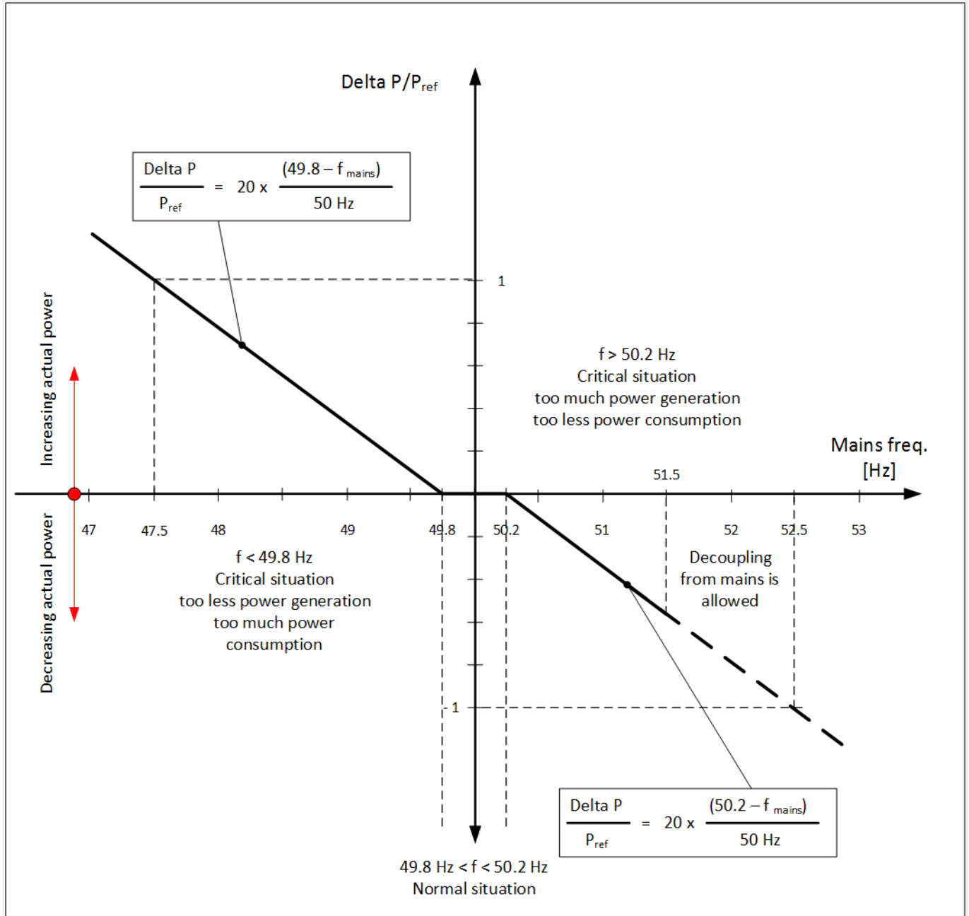
Fig. 128: Dépassement/Surclassement de la consigne de la puissance active pour la stabilisation du réseau
