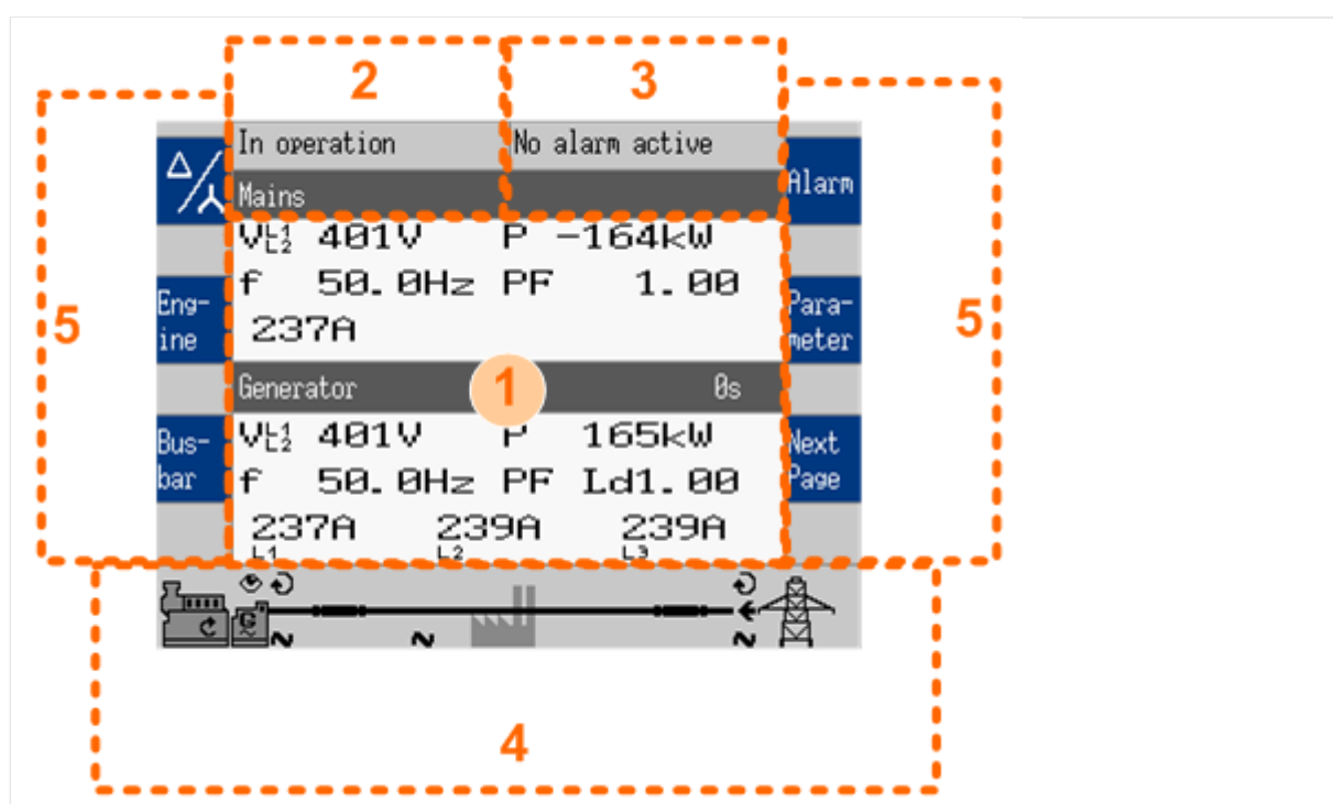
Fig. 88: Écran principal (affiché avec les paramètres par défaut de configuration d'écran)
