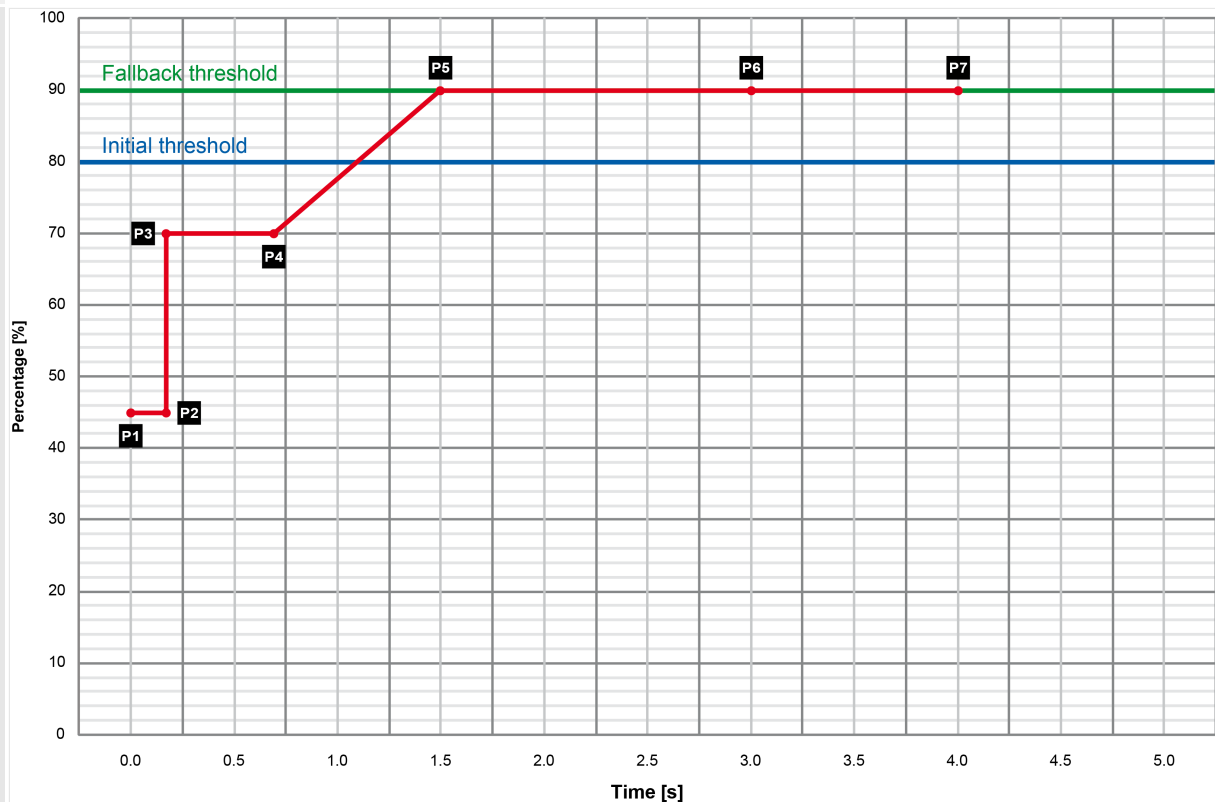
Fig. 141: Courbe de surveillance de tension temporaire
