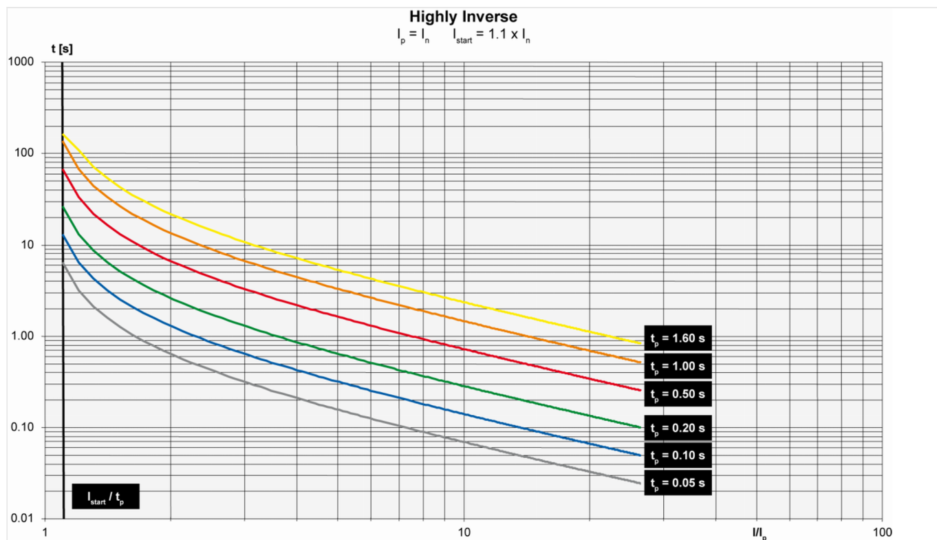
Fig. 130: Caractéristique « très inverse »
