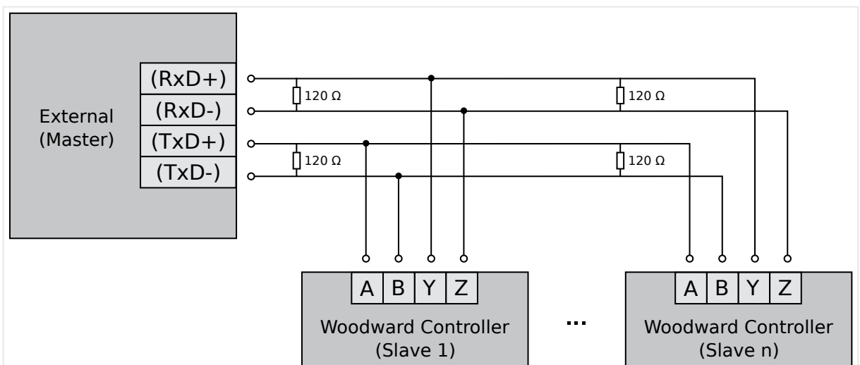
Fig. 78: RS-485 - connexion pour un fonctionnement en duplex intégral
