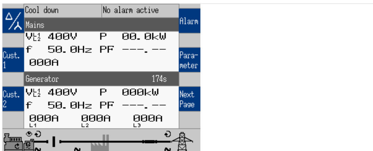
Fig. 112: Affichage de la durée en fonction de la condition de fonctionnement
