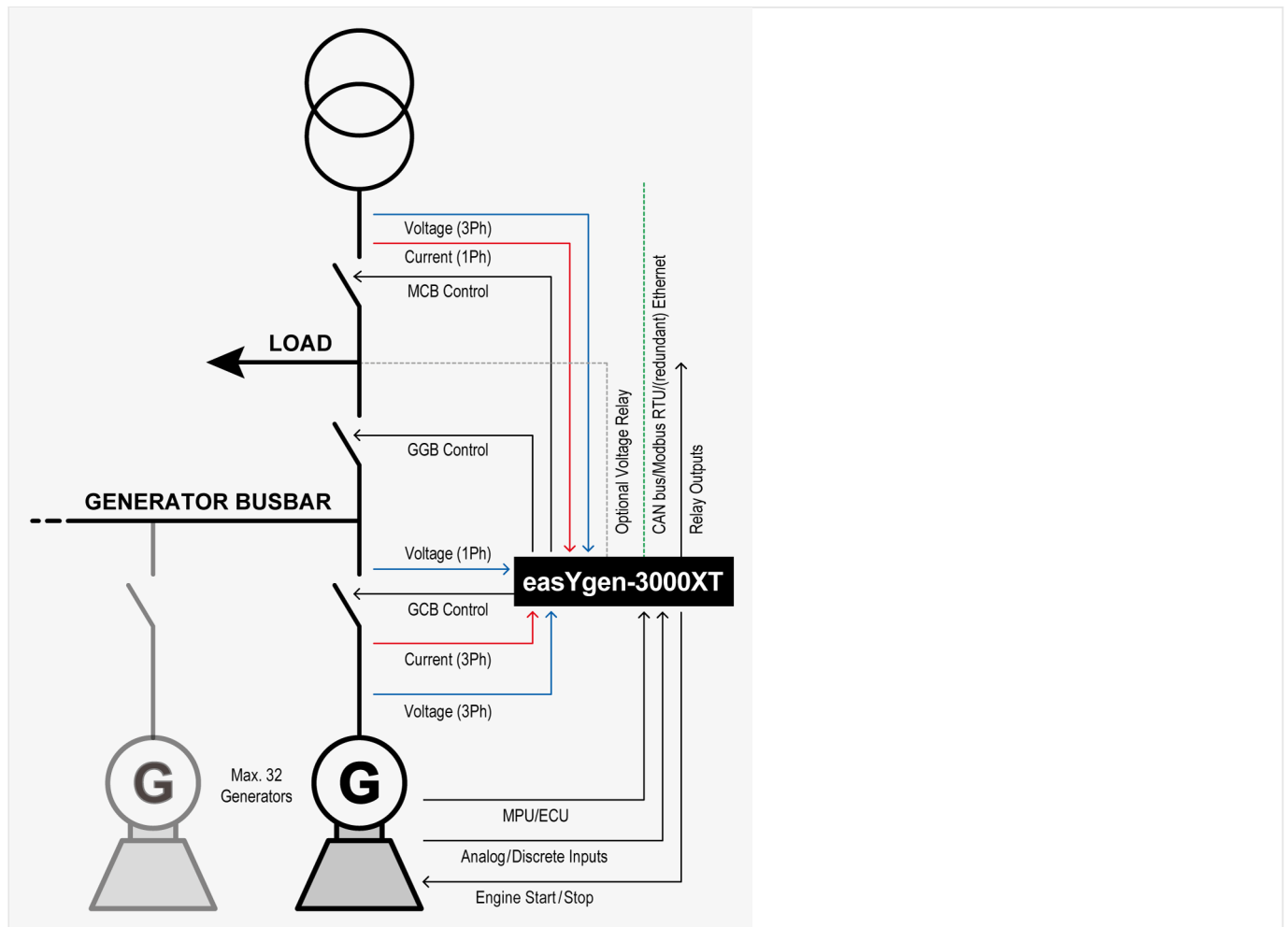
Fig. 1: Configuration d'application type
