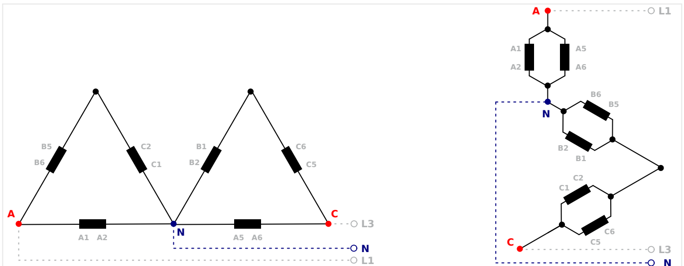
Fig. 31: Enroulements pour générateur- 1Ph 3F
