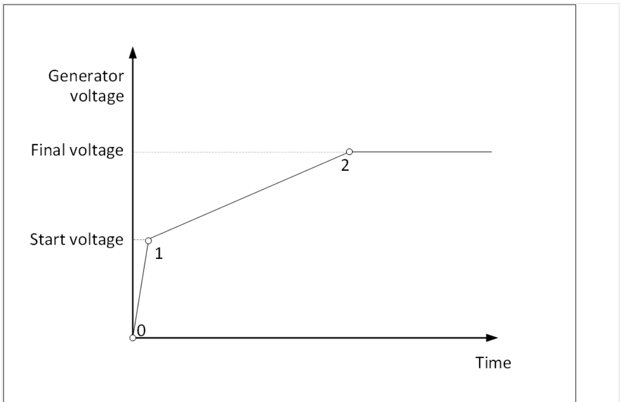
Fig. 118: La séquence de démarrage progressif de l'AVR
