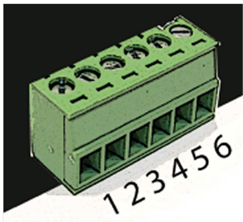
Fig. 76: Connecteur à 6 bornes vissables - RS-485
