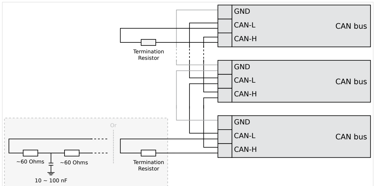
Fig. 81: Terminaison du bus CAN
