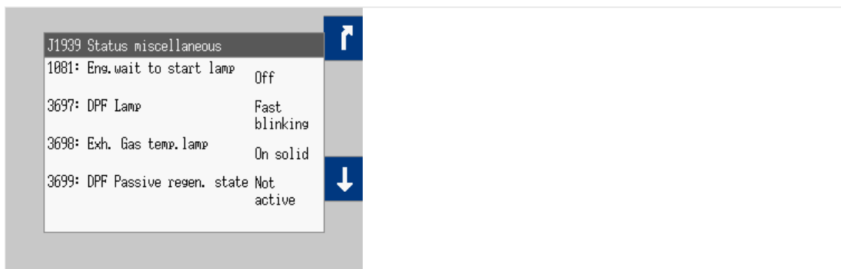
Fig. 111: État J1939 (divers) Écran 1
