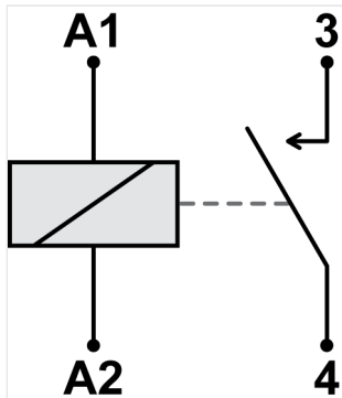
Fig. 113: Contacts normalement ouverts - schéma
